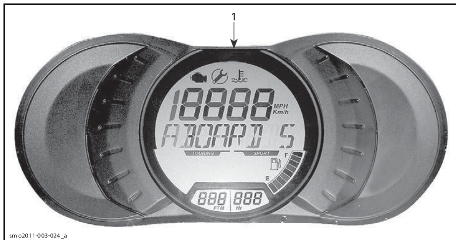
ТИПОВОЙ ВАРИАНТ – МОДЕЛИ GTS 1. Многофункциональная панель приборов
