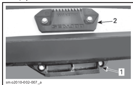
КРЕПЕЖНЫЕ КРОНШТЕЙНЫ ДЛЯ ДЕРЖАТЕЛЯ ВЕЙКБОРДА
