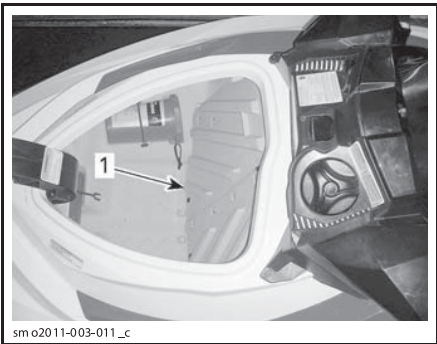
ДОСТУП К ПРЕДОХРАНИТЕЛЮ И АКБ, НОСОВОЕ БАГАЖНОЕ ОТДЕЛЕНИЕ 1. Панель доступа к аккумуляторной батарее
