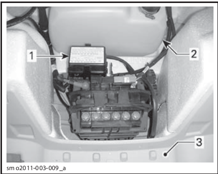
ТИПОВОЙ ВАРИАНТ 1. Блок предохранителей 2. Топливный бак 3. Носовое багажное отделение (панель доступа снята)
