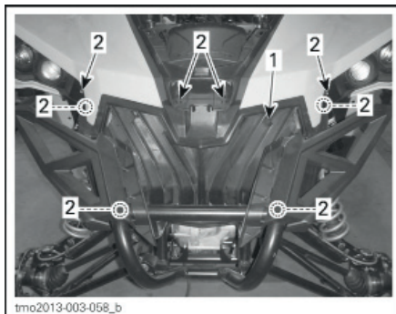
ТИПОВОЙ ВАРИАНТ 1. Пластиковая крышка радиатора 2. Болты
