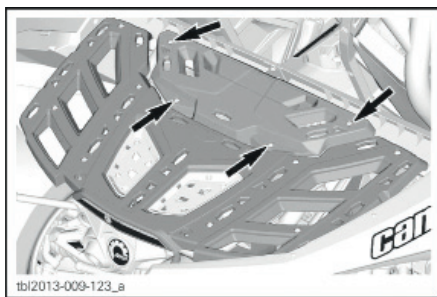
ВОЗДУХОВОДЫ ВАРИАТОРА
