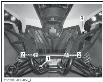
ТИПОВОЙ ВАРИАНТ 1. Нижний болт 2. Верхние болты 3. Бампер
