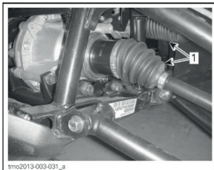
ПЕРЕДНЯЯ ЧАСТЬ МОТОВЕЗДЕХОДА 1. Пыльник внутреннего шарнира приводного вала
