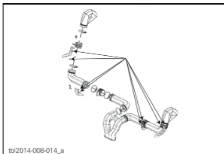
ВОЗДУХОВОДЫ ВАРИАТОРА
