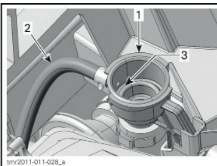
1. Горловина для заправки системы охлаждения 2. Шланг расширительного бачка 3. Уровень жидкости в системе охлаждения (посадочная поверхность крышки радиатора)
