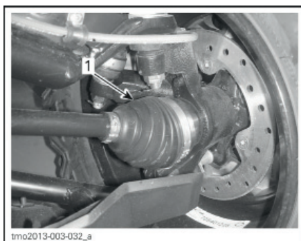
ПЕРЕДНЯЯ ЧАСТЬ МОТОВЕЗДЕХОДА 1. Пыльник наружного шарнира приводного вала
