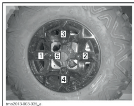
ПОСЛЕДОВАТЕЛЬНОСТЬ ЗАТЯЖКИ – ТИПОВОЙ ВАРИАНТ
