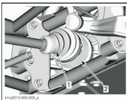
ЗАДНЯЯ ЧАСТЬ МОТОВЕЗДЕХОДА (КОМПОНЕНТЫ СНЯТЫ ДЛЯ НАГЛЯДНОСТИ) 1. Пыльник внутреннего шарнира приводного вала 2. Теплоотвод
