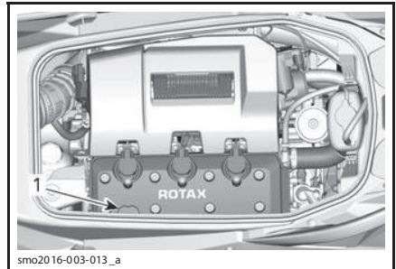
1. Расположение крышки маслoзаливной горловины
