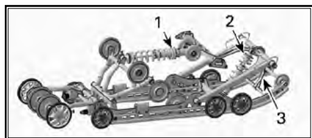
ЗАДНЯЯ ПОДВЕСКА PPS-6900-F2
