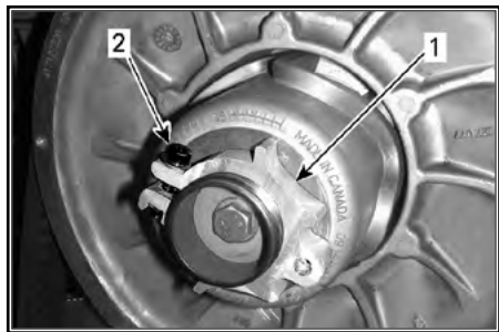
РЕГУЛИРОВОЧНАЯ МУФТА
