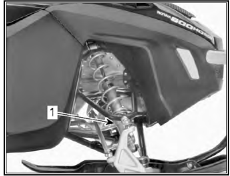
ТИПОВОЙ ВАРИАНТ — РЕГУЛЯТОР КУЛАЧКОВОГО ТИПА
