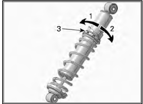
РЕГУЛЯТОР КУЛАЧКОВОГО ТИПА — АМОРТИЗАТОР НРР
