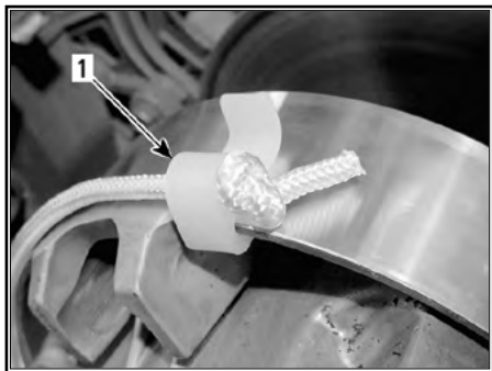
1. Расположение зажима
