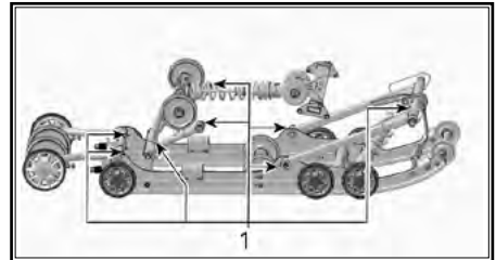
1. Пресс-масленки
